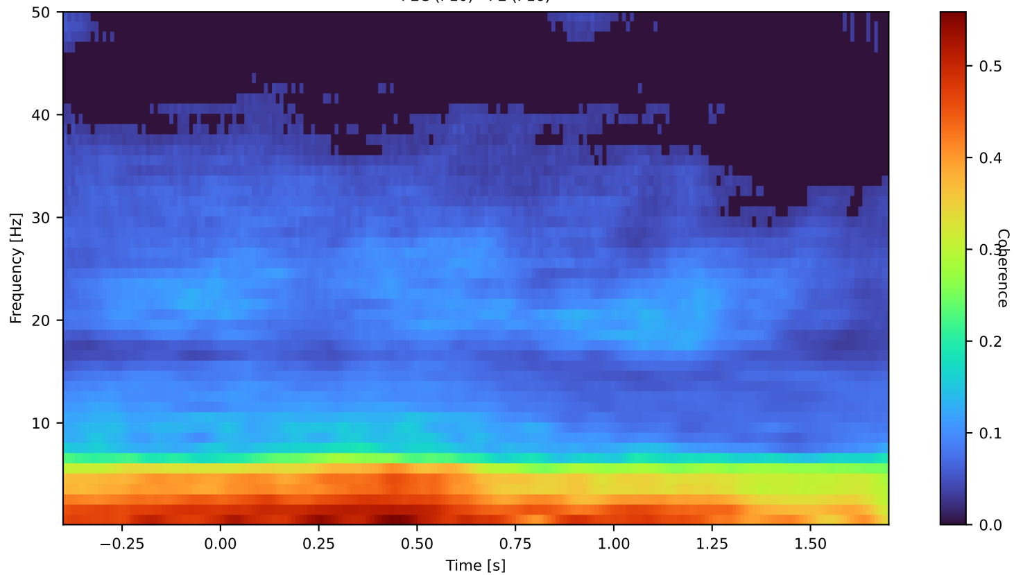
PEC (P10) - PE (P16)
